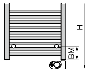
Detailzeichnung elektrisch
