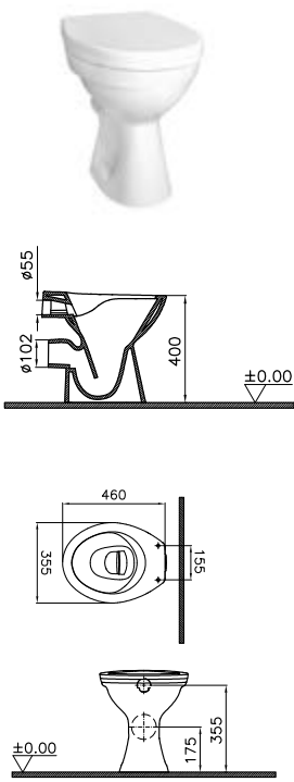
DIANA O100 Tiefspül-Stand-WC** spülrandlos mit waagrechtm Abgang, Ausladung 460 mm, (DI000601001)
