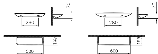
DIANA O100 Aluminium Einlegerost
