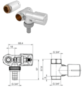
DIANA O100 Nebenanschlussventil für Wandbatterien, mit Rückflussverhinderer und Schlauchverschraubung, poliert verchromt, mit Distanzstück zur Montage von Wandbatterien, Anschluss links, (DI407945500)
