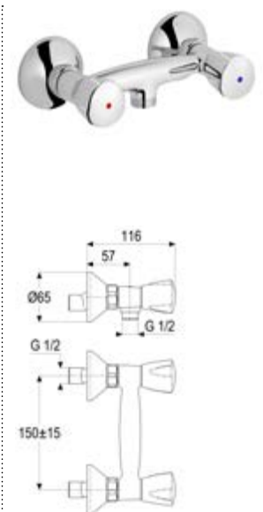
DIANA O100 Wannenarmatur eigensicher ohne Brausegarnitur, verchromt, (DI407402500)
